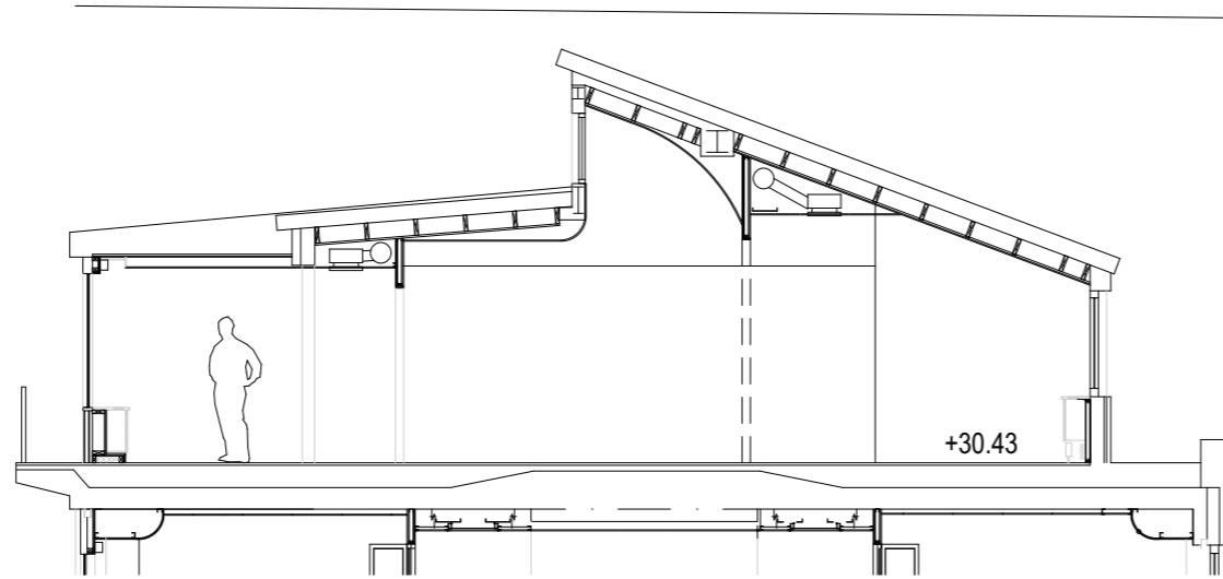
SEKTION A - 1:100
